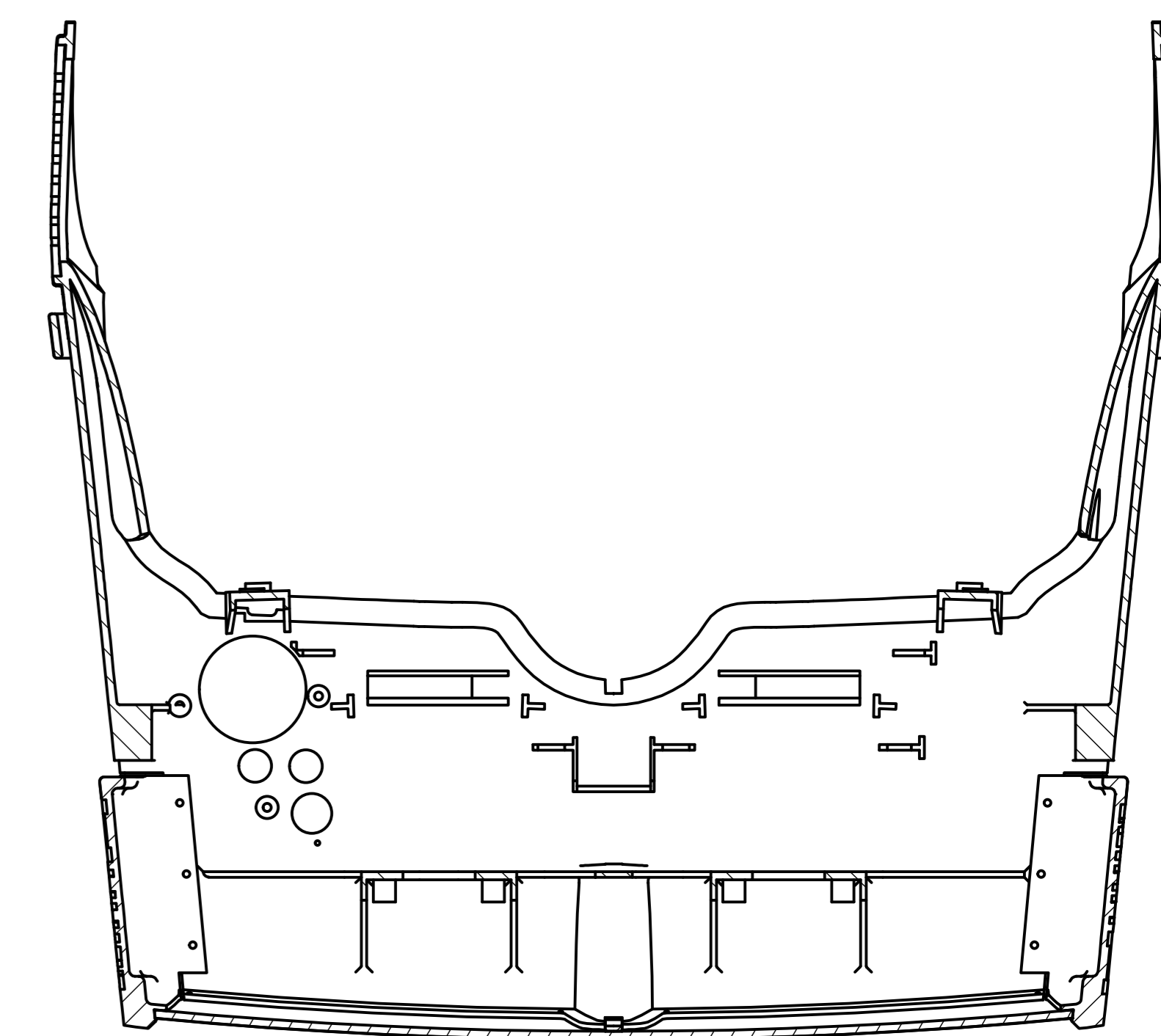
SECTION A-A SCALE 1 : 1
